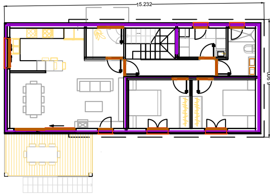
PLANTA BAIXA
