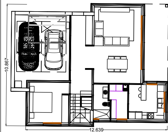
PLANTA BAIXA
