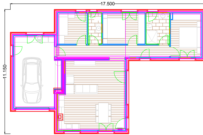
PLANTA BAIXA
