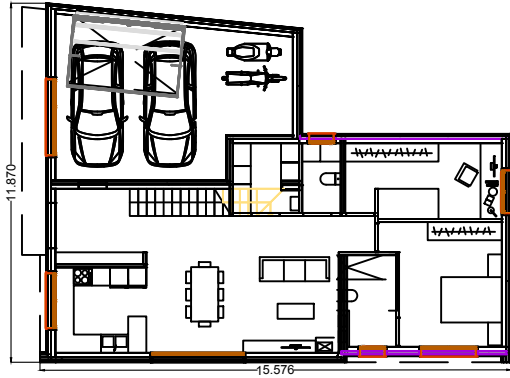
PLANTA BAIXA
