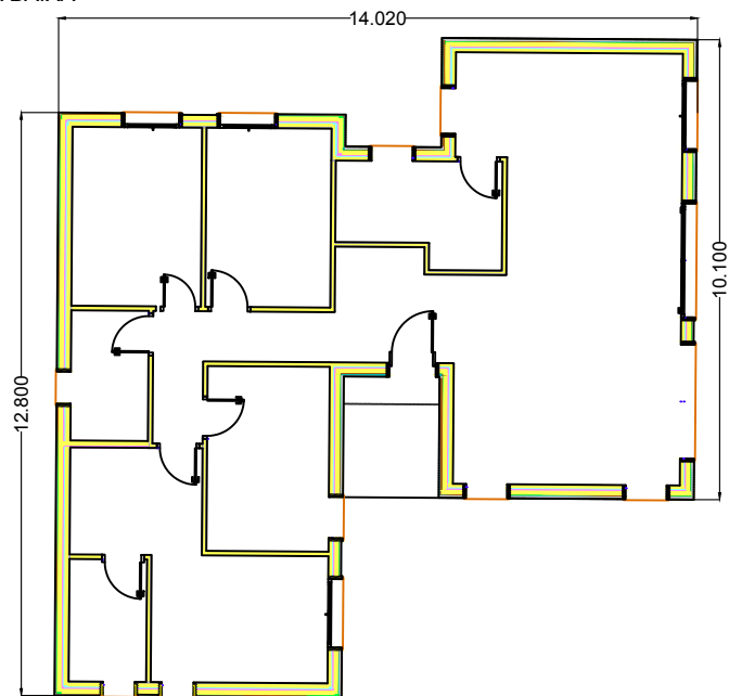
PLANTA BAIXA
